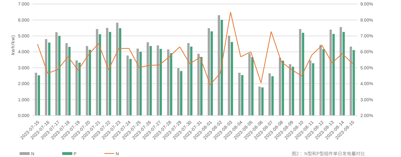
图2：N型和P型组件单日发电量对比
